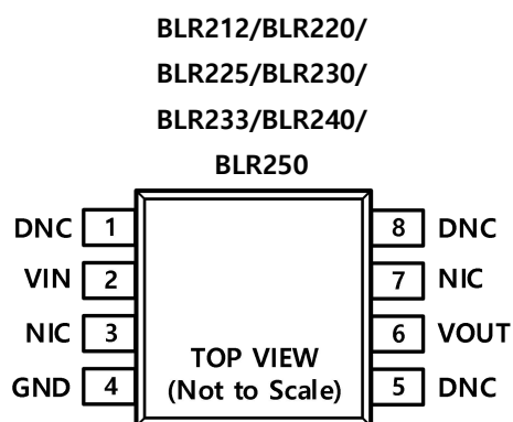
图 1.1 8 引脚 SOIC
