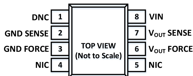
图 1.2 8 引脚 MSOP
