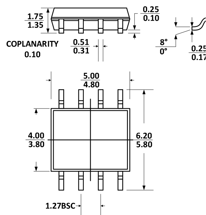
图 31.1 8 引脚标准小型封装[SOIC_N]图示尺寸单位：毫米
