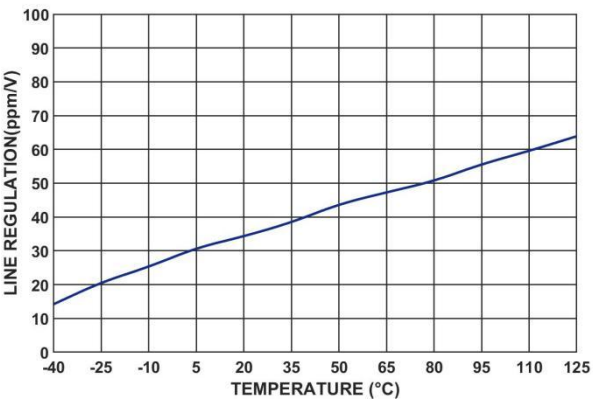
图 17 BLR230 电压调整率与温度的关系
