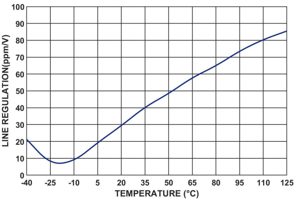
图 23 BLR240 电压调整率与温度的关系
